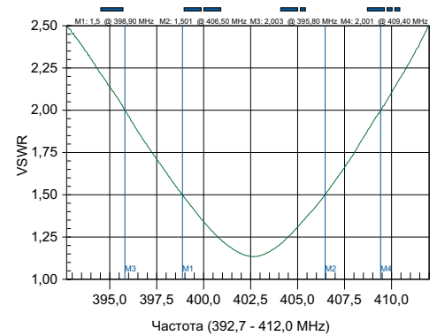
График КСВ А-300МУ-N
